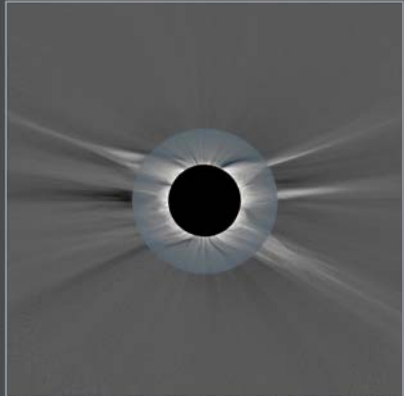
Total Solar Eclipse 2006 © 2006 Václav Rulík, Hana Druckmüllerová, Miloslav Druckmüller, SOHO ESA/NASA
